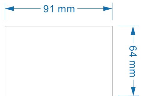
显示面板开孔尺寸图
